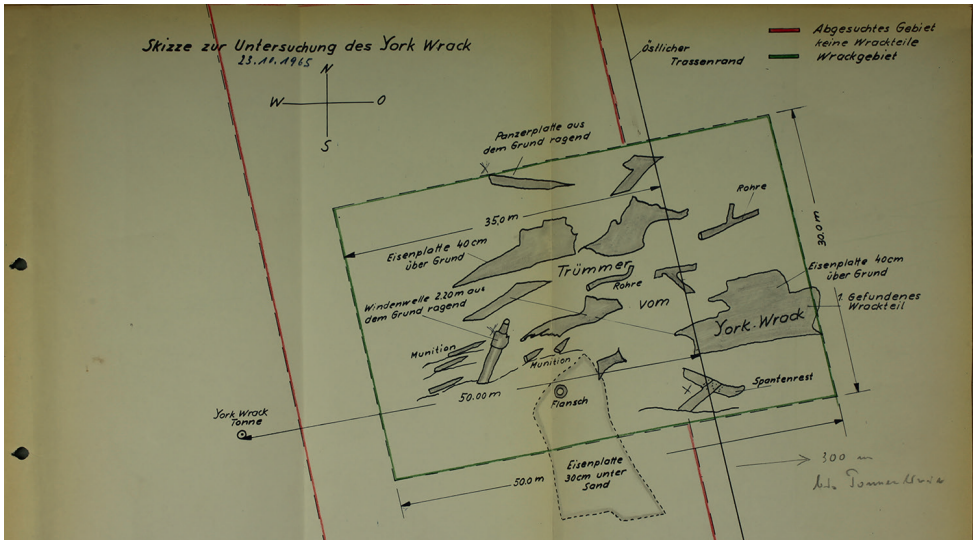
Abb. 3: Skizze der Untersuchung des Wracks von SMS York (NLA OL, Rep 680 WHV Best. 238-23 Nr. 587)
